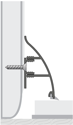
Przykład montażu
