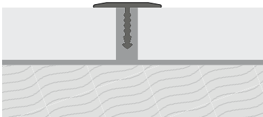
Przykład montażu
