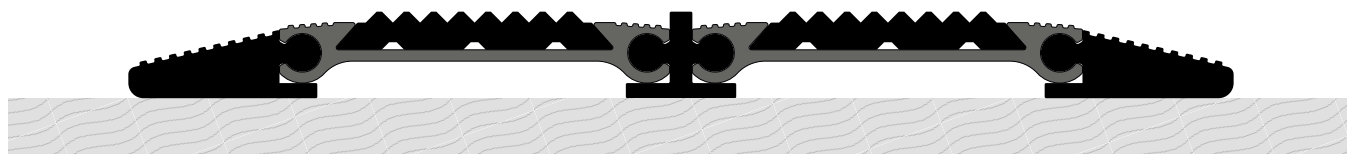
Przykład systemu samodzielnego dla wykładziny dywanowej
