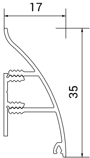
Przekrój profilu
