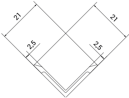
Przekrój profilu
