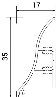
Przekrój profilu
