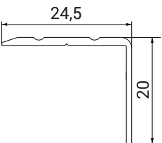
Przekrój profilu
