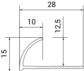
Przekrój profilu
