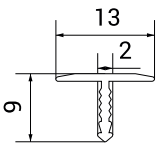
Przekrój profilu
