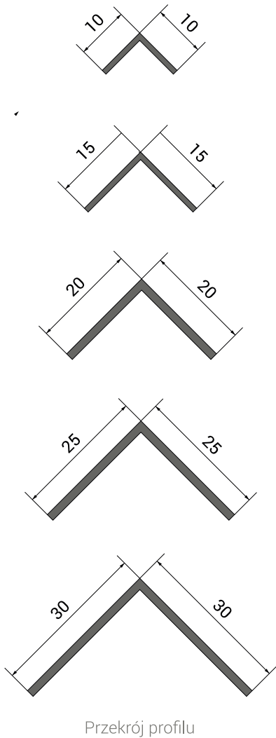
Przekrój profilu
