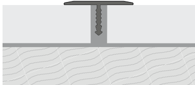
Przykład montażu
