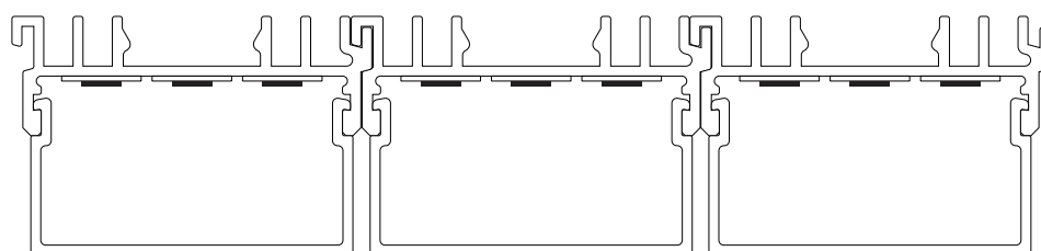
Exemple de montage
