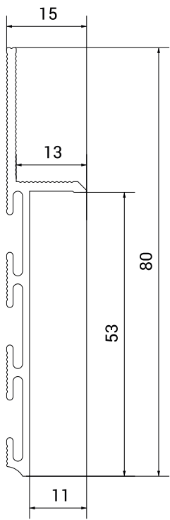
Przekrój profilu
