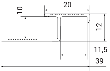
Przekrój profilu
