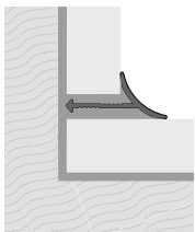
Przykład montażu
