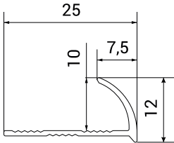
Przekrój profilu
