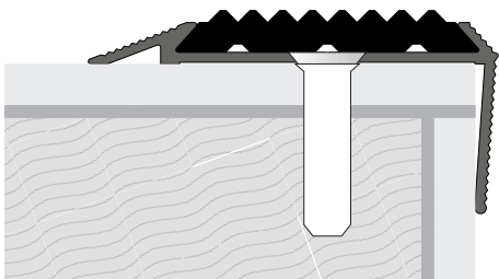
Przykład montażu
