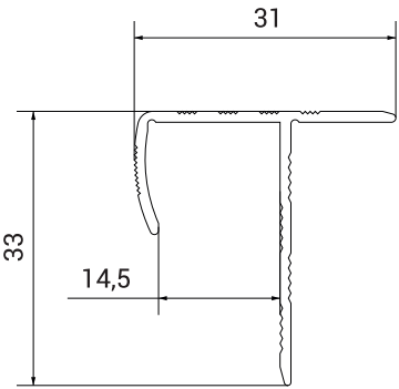
Przekrój profilu
