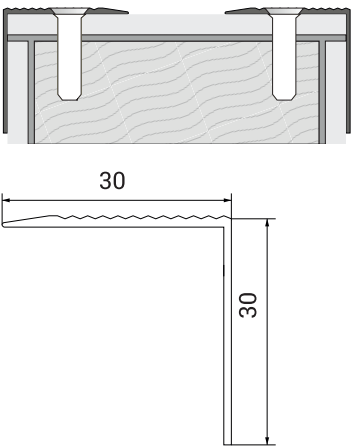
Przekrój profilu
