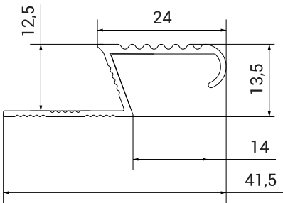
Przekrój profilu
