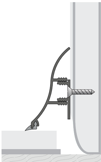
Przykład montażu
