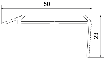
Przekrój profilu
