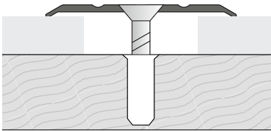
Przykład montażu
