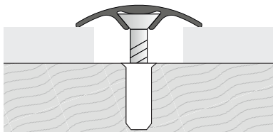
Przykład montażu
