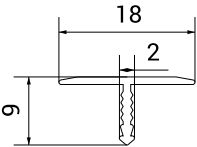
Przekrój profilu
