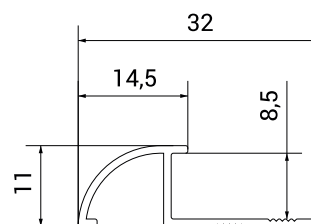
Przekrój profilu
