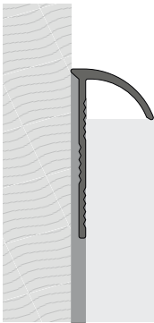
Przykład montażu
