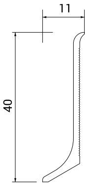
Przekrój profilu
