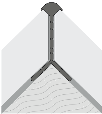
Przykład montażu
