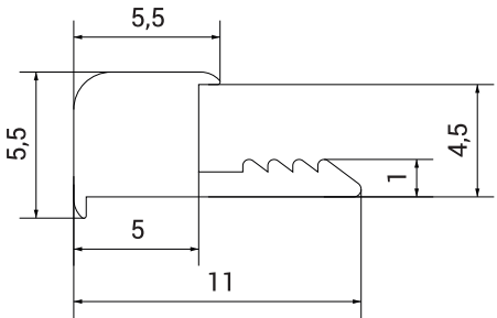
Przekrój profilu
