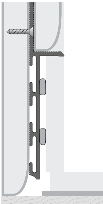
Przykład montażu
