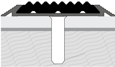
Przykład montażu
