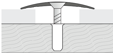
Przykład montażu
