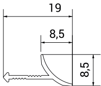
Przekrój profilu
