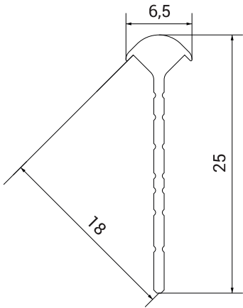
Przekrój profilu
