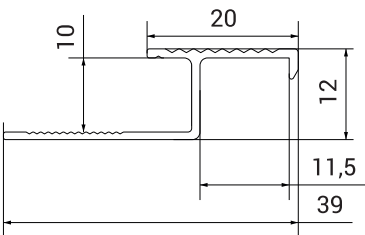
Схема профілю
