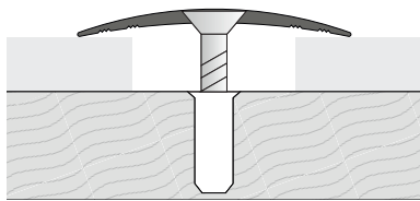
Приклад монтажу
