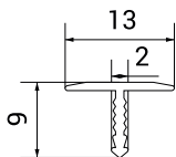
Схема профілю
