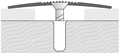
Приклад монтажу
