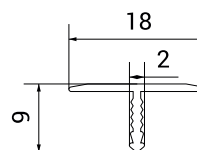
Схема профілю
