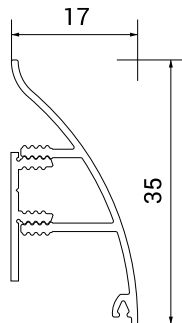
Схема профілю
