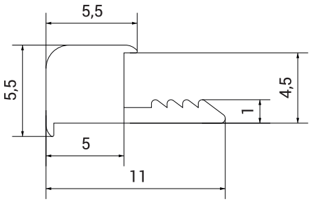
Схема профілю
