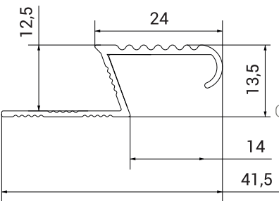
Схема профілю
