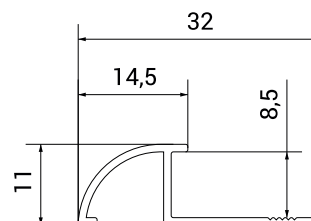
Схема профілю
