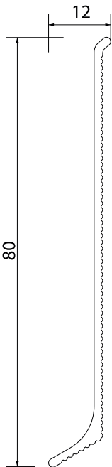
Схема профілю
