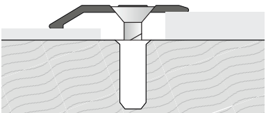
Приклад монтажу
