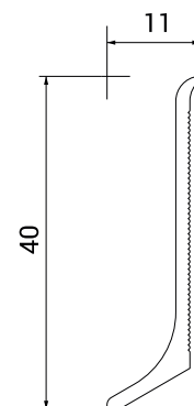
Схема профілю
