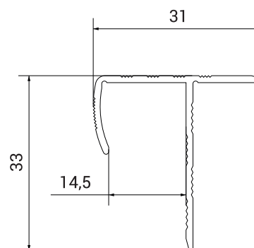
Схема профілю
