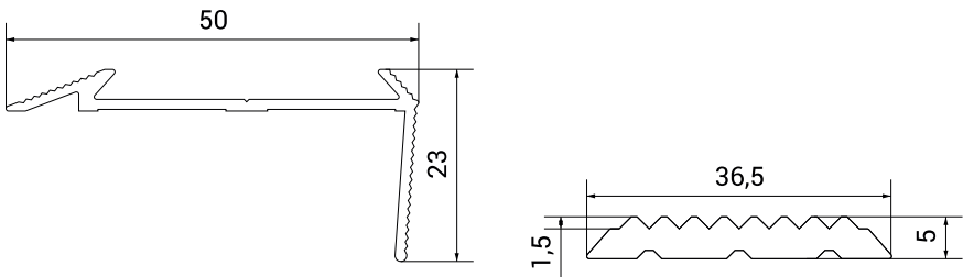
Схема профілю
