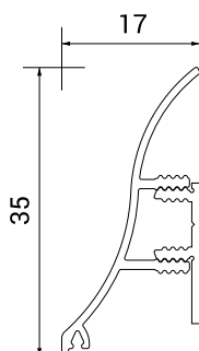
Схема профілю
