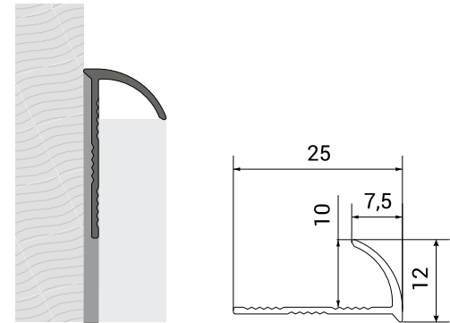
Приклад монтажу Схема профілю
