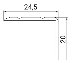
Схема профілю
