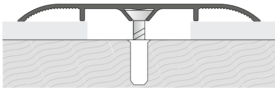
Приклад монтажу
