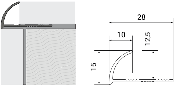
Приклад монтажу Схема профілю
