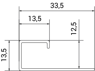
Схема профілю
