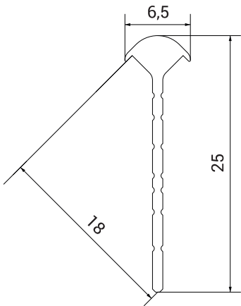
Схема профілю
