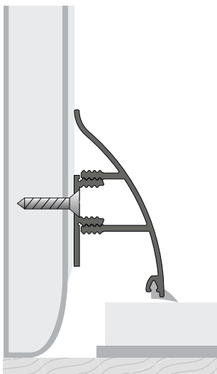
Приклад монтажу
