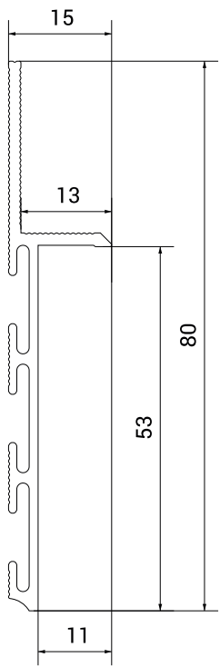
Схема профілю
