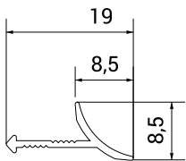
Схема профілю
