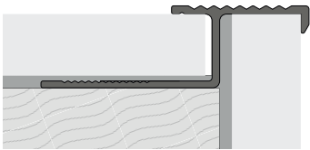
Приклад монтажу
