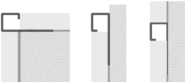
Приклад монтажу
