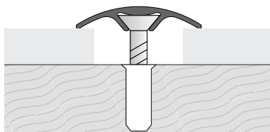
Приклад монтажу
