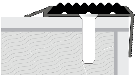
Приклад монтажу
