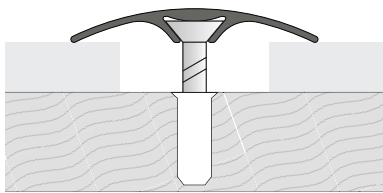
Приклад монтажу
