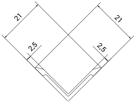
Схема профілю
